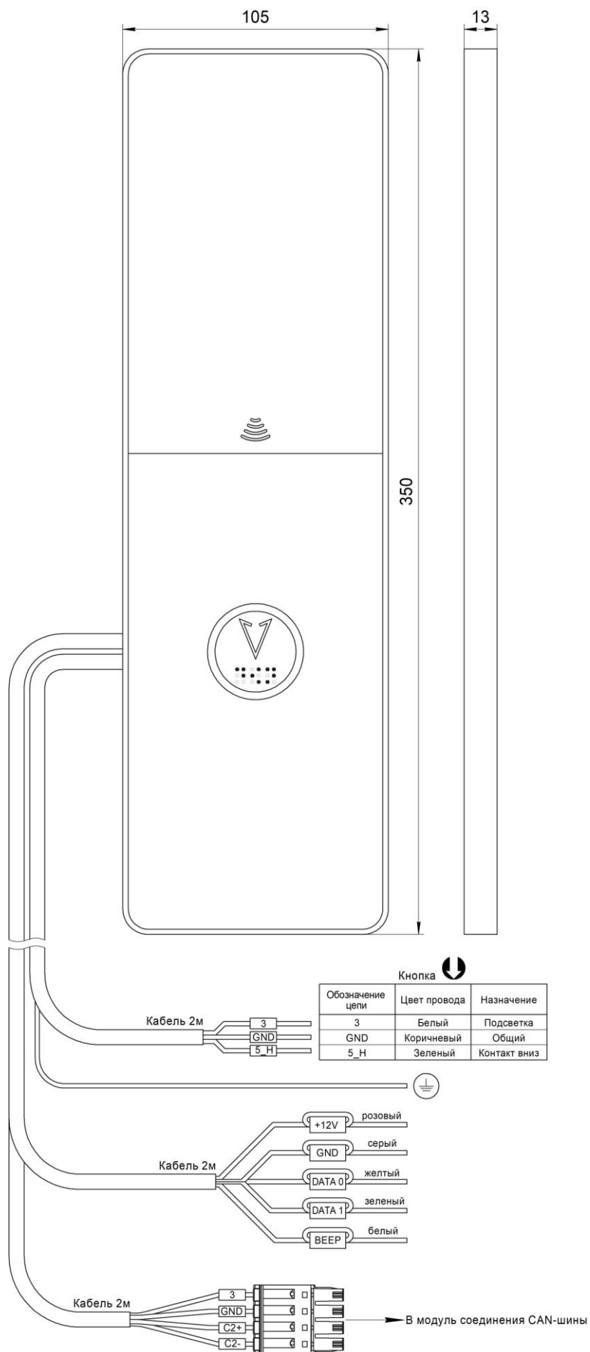
Рис.1 Внешний вид, габаритные и установочные размеры Вызывного поста МАЛАХИТ НШЕК.468381.015-19
